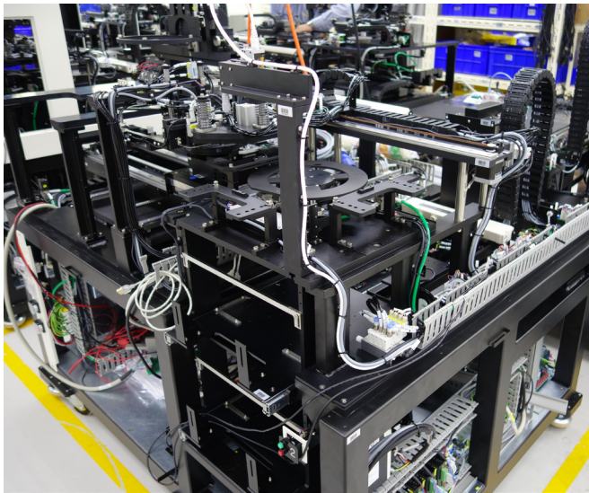
Сборка зондовой установки MPI Assembly of MPI's probe system
